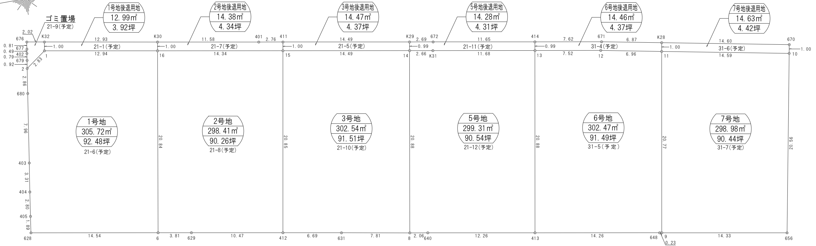
座 標 求 積 表
